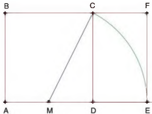
FIGURA 1.3 Rectángulo áureo
